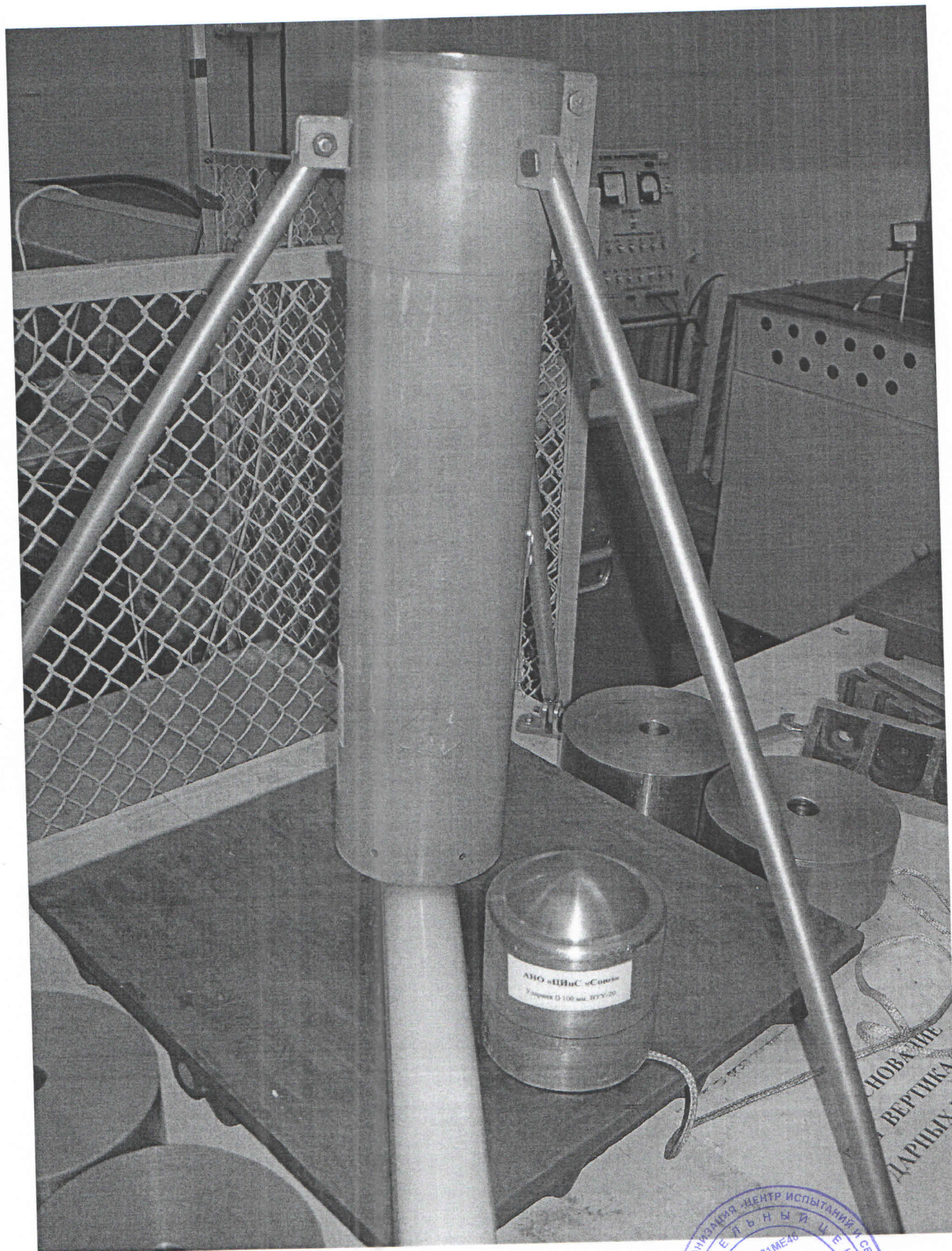
Рис. 3 Вид на вертикальное ударное устройство ВУУ-20 с ударником D-100 мм перед испытаниями.
